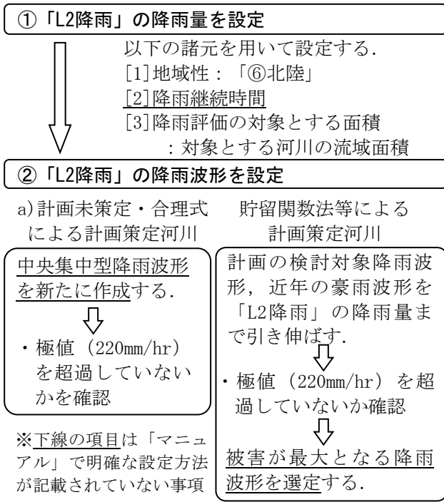
図-2 「L2降雨」の降雨量・降雨波形設定の主な流れ
