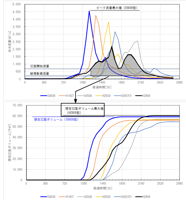
図-5 降雨波形毎のピーク流量(上段)・想定氾濫量(下段)の算定例
