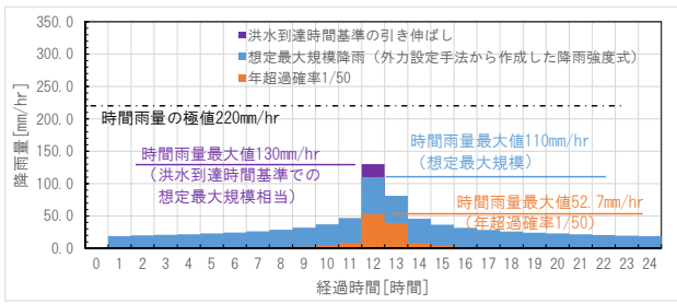
図-4 「L2降雨」計算例(3) (10分刻みでの雨量を毎正時で合算した値)
