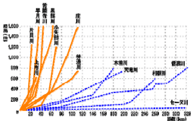
図-1 河川縦断概略図 5)
