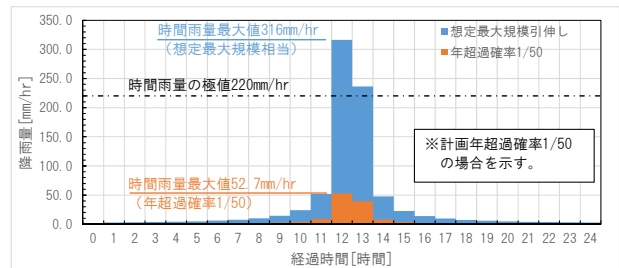
図-3 「L2降雨」計算例(1)
